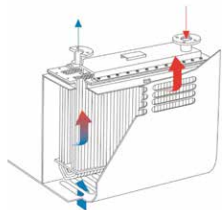
longitudinal installation
